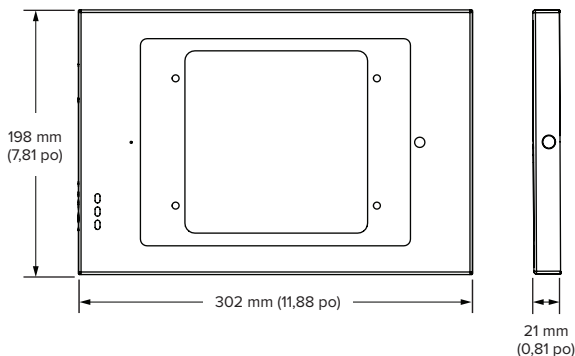
Boîtier
